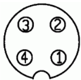
Belegung des Steckers (Sicht auf Stifte/Einbaustecker male)
